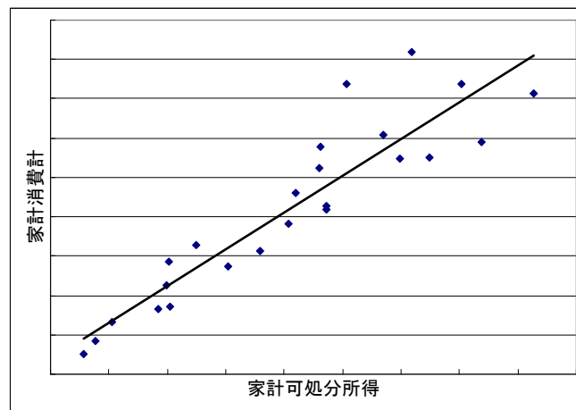
図 3-1 散布図と回帰方程式
